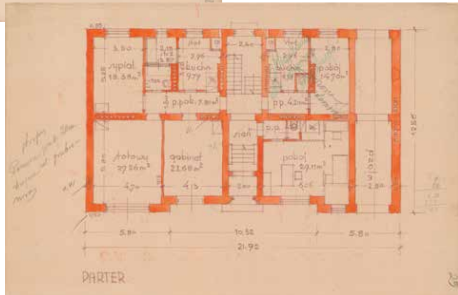
Projekt budowy domu mieszkalnego przy ulicy Mickiewicza, autorstwa Kazimierza Prokulskiego, 1938 rok.
