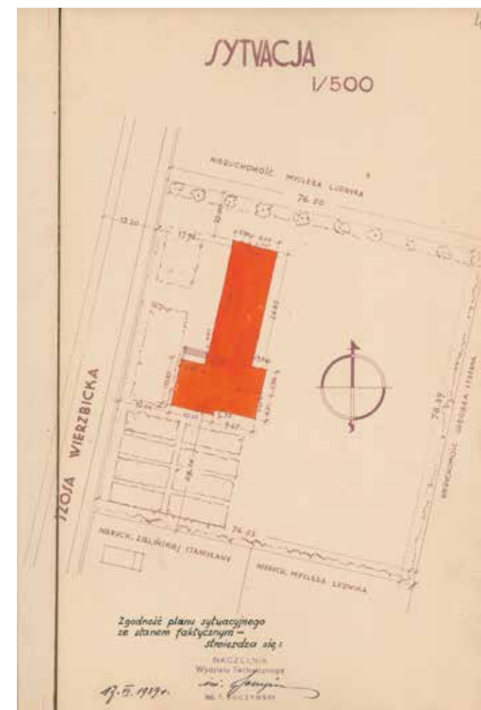
Szkoła powszechna, murowana przy ulicy Wierzbickiej na przedmieściu Żakowice według projektu Józefy Mehl, 1939 rok.
