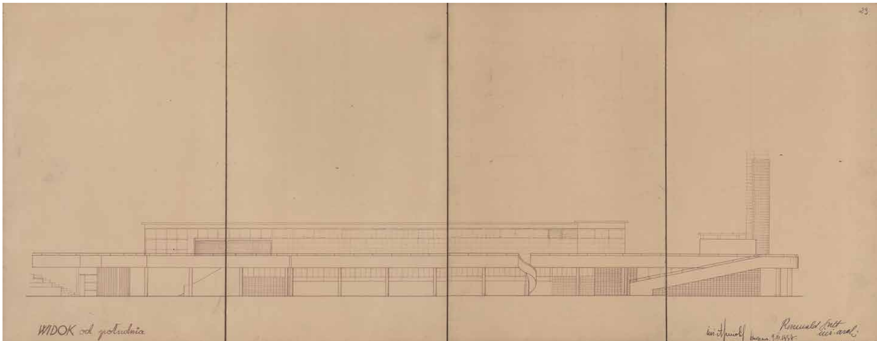
Projekt pływalni na stadionie im. Marszałka Piłsudskiego według architekta Romualda Gutta, 1937 rok.
