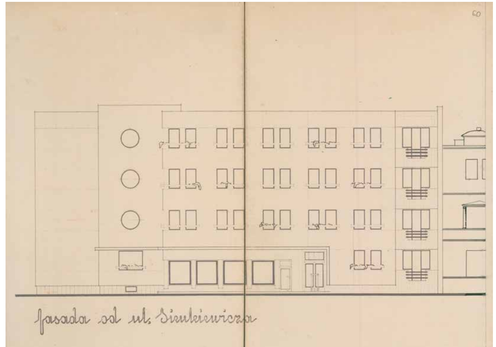
Projekt budowy domu na posesji u zbiegu ulic Moniuszki i Sienkiewicza według Artura Hasklera, 1938-1939 rok.
