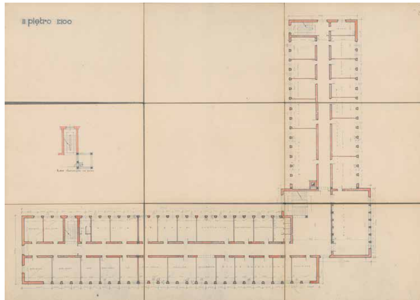
Projekt gmachu Dyrekcji Lasów Państwowych w Radomiu przy zbiegu ulic Świeżej (obecnie Kelles-Krauz) i ulicy 1 Maja (obecnie 25 Czerwca) opracowany przez Walerego Sahajdakowskiego pod kierownictwem Jana Ludwika Zabłockiego w 1937 roku.
