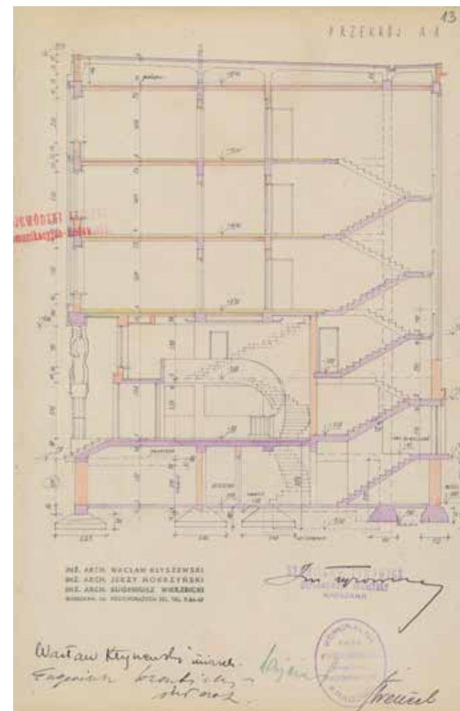
Projekt gmachu Komunalnej Kasy Oszczędności na Placu Konstytucji 3 Maja 4, autorstwa Stanisława Tyrowicza i zespołu architektów „Tygrysy”: Wacława Kłyszewskiego, Jerzego Mokrzyńskiego, Eugeniusza Wierzbickiego, 1939 rok.
