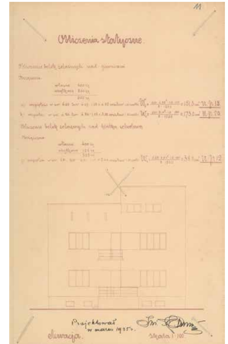
Projekt domu murowanego Zofii Gmyrkowej przy ulicy Mickiewicza 11 (obecnie Mickiewicza 9), Alfons Pinno, 1935 rok.
